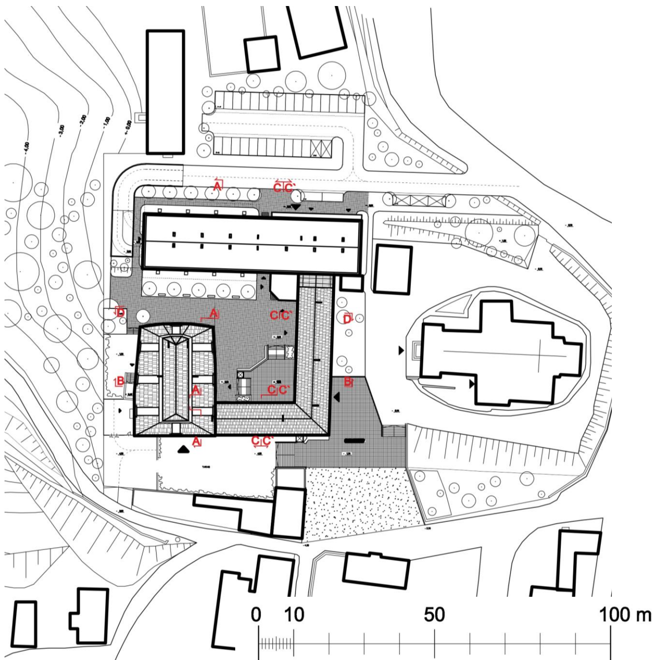
il. 79 Zespół zamkowy w Ujeździe Śląskim. Sytuacja. Koncepcja zagospodarowania terenu.
