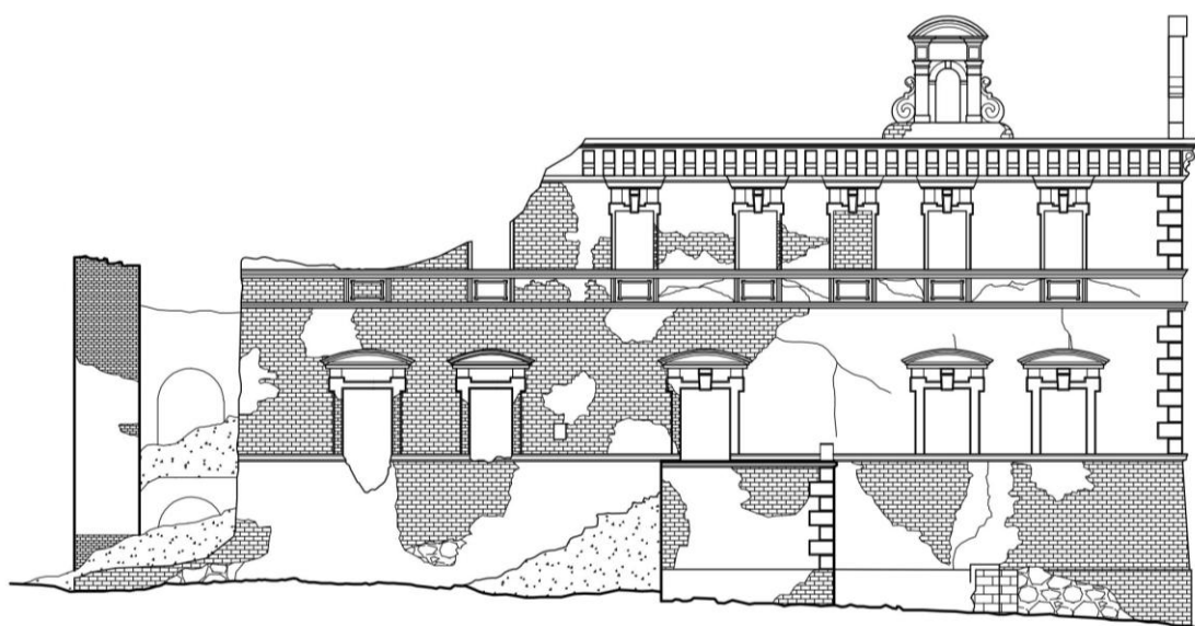
il. 49 Skrzydło zachodnie. Elewacja zachodnia. [(opracowanie autorskie) na podstawie poz.04]
