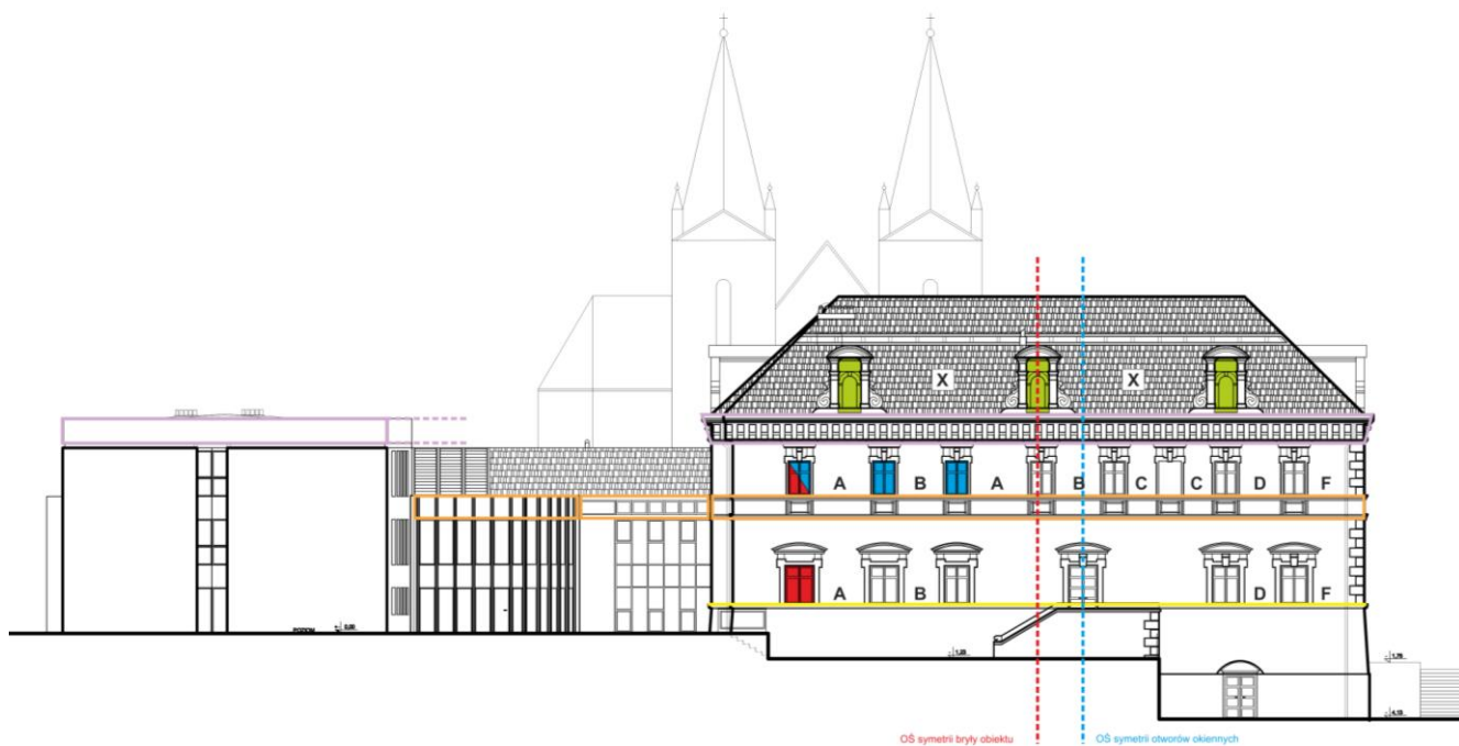
il. 82 Elewacja zachodnia.
