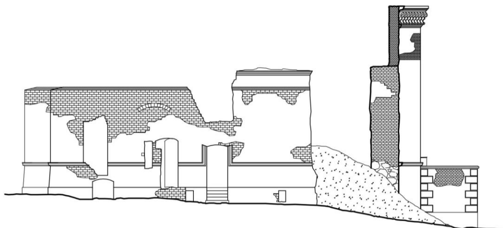
il. 56 Skrzydło zachodnie. Elewacja północna. [(opracowanie autorskie) na podstawie poz.04]
