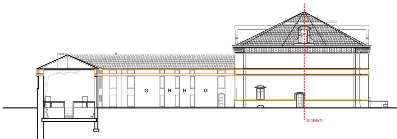
il. 83 Przekrój DD z widokiem na północną elewację zachodniego i południowego skrzydła.
