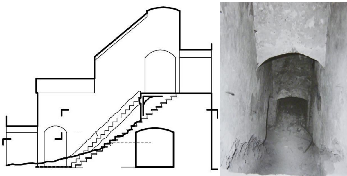
il. 62 Skrzydło zachodnie. Jednobiegowa klatka schodowa – pomieszczenie 1/8 z zaznaczonymi przebudowami biegu. [(opracowanie autorskie) na podstawie poz.04]
