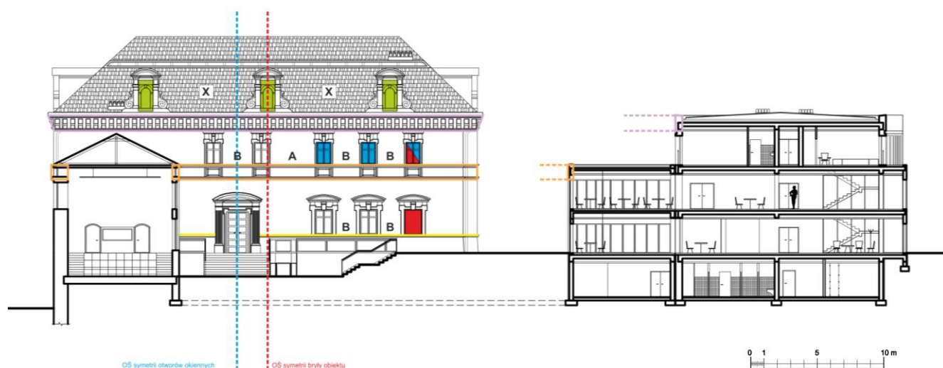
il. 81 Przekrój CC z widoczną wschodnią elewacją zachodniego skrzydła.
