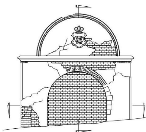
PORTAL NR.2/BUD.WSCHODNI WIDOK
