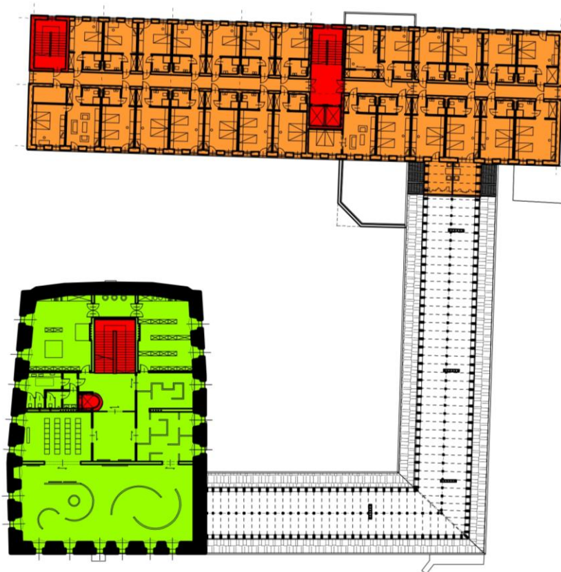
il. 90 Rzut kondygnacji +1 (skrzydło północne - rzut kondygnacji +2)
