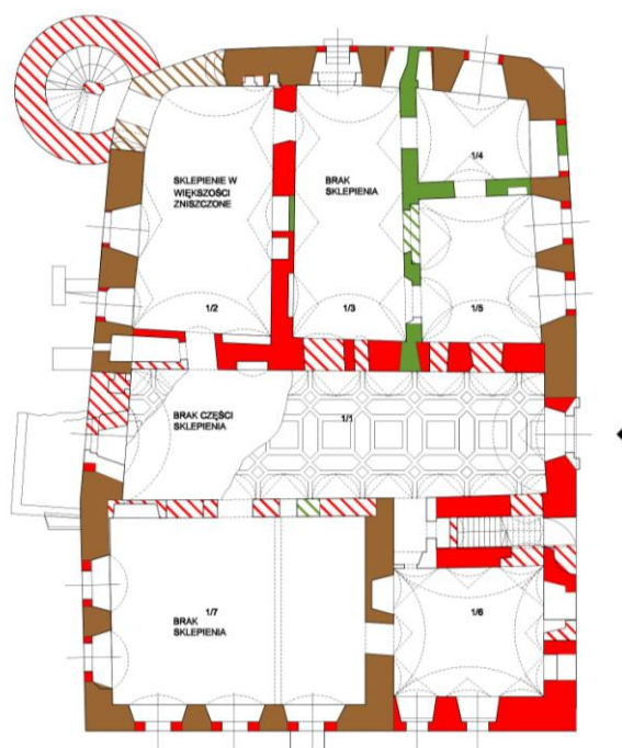
RZUT PARTERU - założenie sklepienia (stan tech. z 1978r.)
