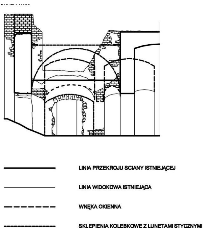
il. 75 Skrzydło zachodnie. Rozwinięcie pn. ściany pom. 1/3 [(opracowanie autorskie) na podstawie poz.04]
