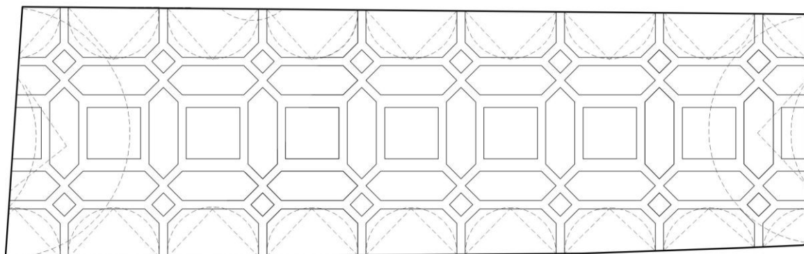
il. 69 Skrzydło zachodnie. Schemat reliefowego ornamentu okuciowego sklepienia sieni , pomieszczenie 1/1. [(opracowanie autorskie) na podstawie poz.04]
