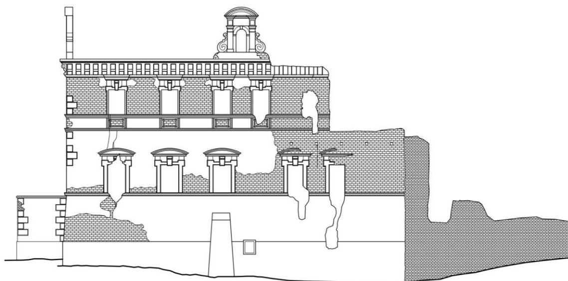
il. 50 Skrzydło zachodnie. Elewacja południowa. [(opracowanie autorskie) na podstawie poz.04]
