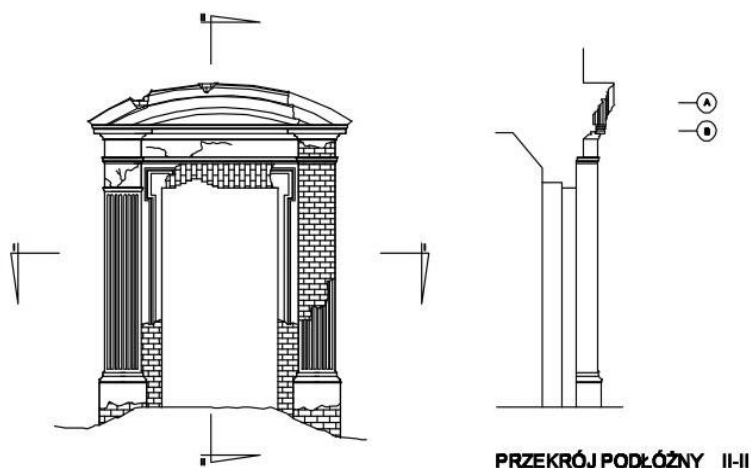
PORTAL NR.1/BUD.WSCHODNI WIDOK Stan techniczny portalu z roku 1978.
