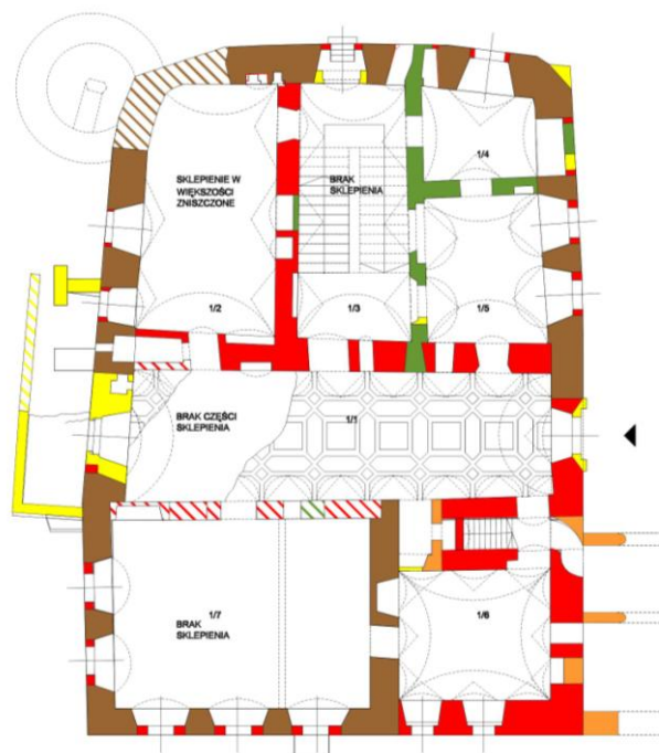
RZUT PARTERU
