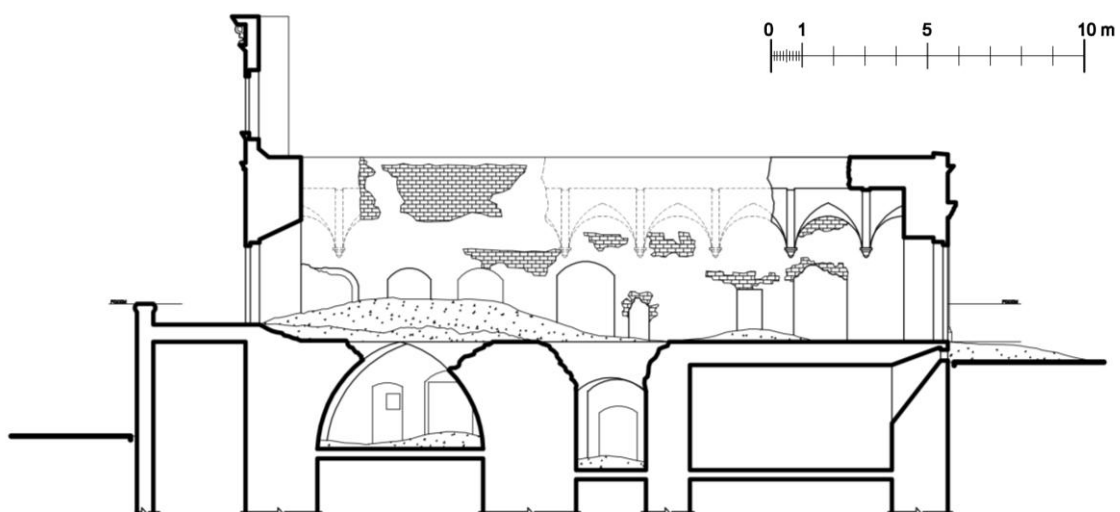
il. 65 Skrzydło zachodnie. Przekrój podłużny A-A [(opracowanie autorskie) na podstawie poz.04]
