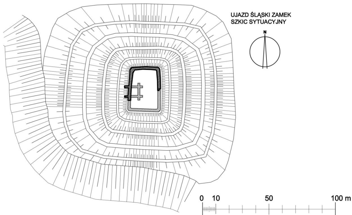
il. 31 Szkic sytuacyjny zamku i obwałowań - Ujazd (koniec XIII w.) [(opracowanie autorskie) na podstawie poz.05]
