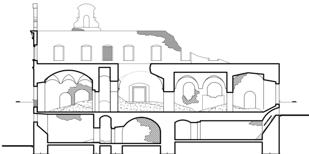
il. 65 Skrzydło zachodnie. Przekrój podłużny A-A [(opracowanie autorskie) na podstawie poz.04]
