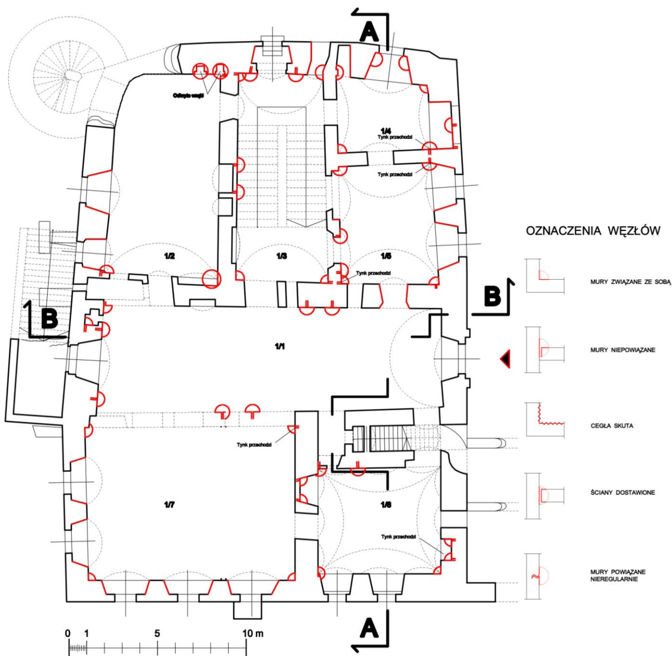
il. 67 Skrzydło zachodnie. Parter. [(opracowanie autorskie) na podstawie poz.04]
