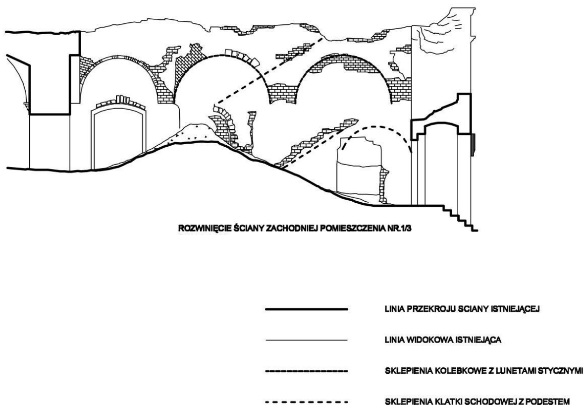
il. 74 Skrzydło zachodnie. Rozwinięcie zachodniej ściany pomieszczenia 1/3.
