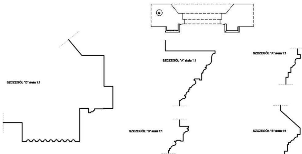
PRZEKRÓJ POPRZECZNY III-III
