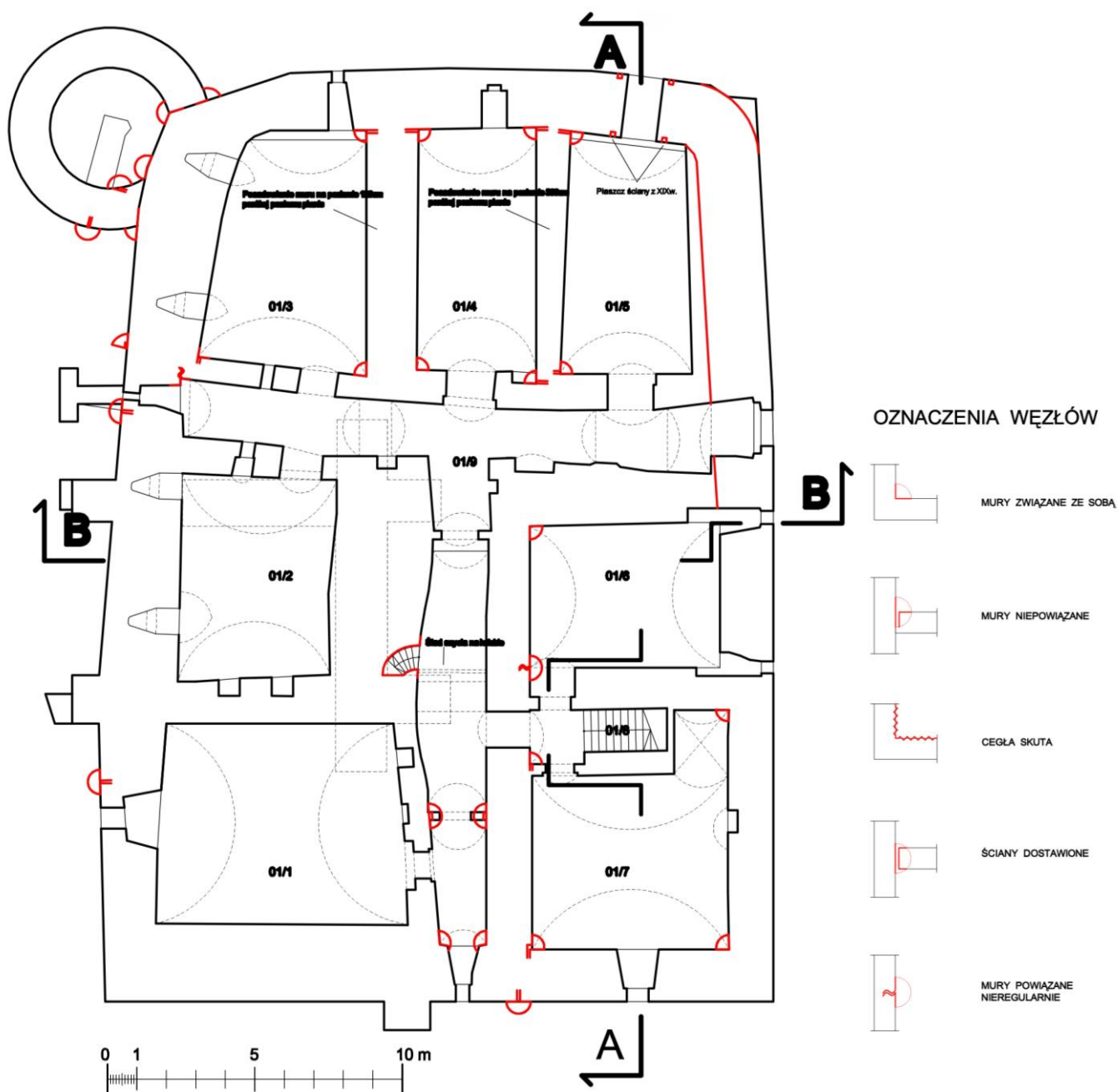
il. 60 Skrzydło zachodnie. Piwnice. [(opracowanie autorskie) na podstawie poz.04]
