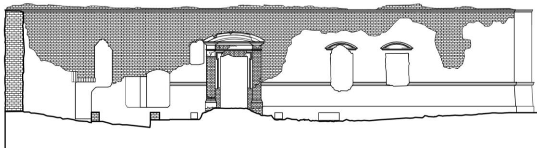
il. 45 Skrzydło zach. Elewacja wsch. (widok z wew. dziedzińca). [(opracowanie autorskie) na podstawie poz.04]
